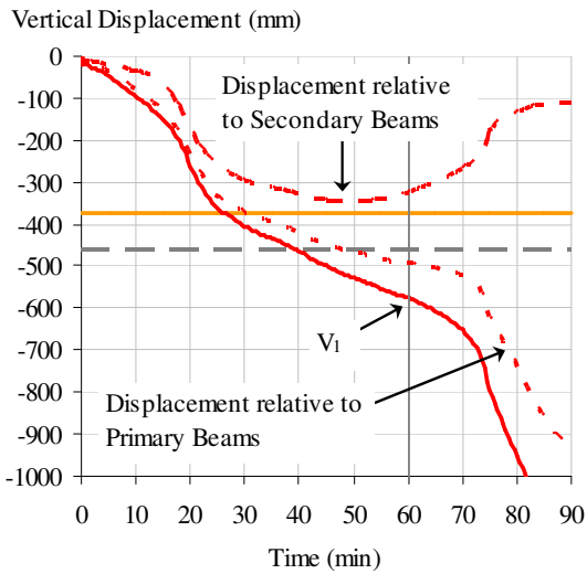
Fig. 7: Vulcan V1 edge beam failure
